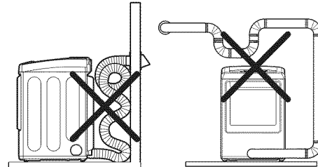
Conduco demasiado largo o muy torcido Tubería demasiado larga o con demasiados codos
