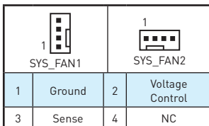
Connecteurs pour ventilateurs en mode DC
