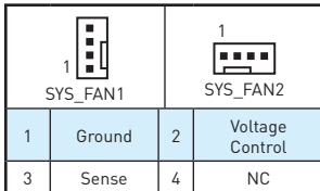
DC 모드 팬 커넥터
