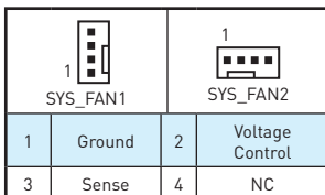
DC 模式風扇電源接頭
