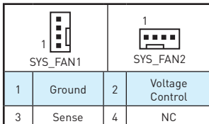
DCモードファンコネクタ
