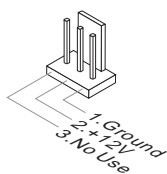
SYSFAN3/ SYSFAN4
