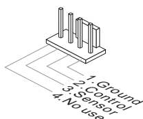
SYSFAN1/ SYSFAN2
