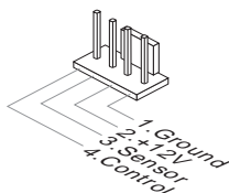
CPUFAN
