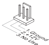
SYSFAN3/ SYSFAN4
