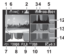
RGB histogram
