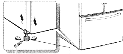
destornillador de punta chata (-) Palanca de control
