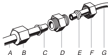
A. Tuyau d'eau dur du réfrigérateur B. Écrou (fourni) C. Renflement D. Raccord (à acheter) E. Virole (à acheter) F. Écrou (à acheter) G. Canalisation du domicile
